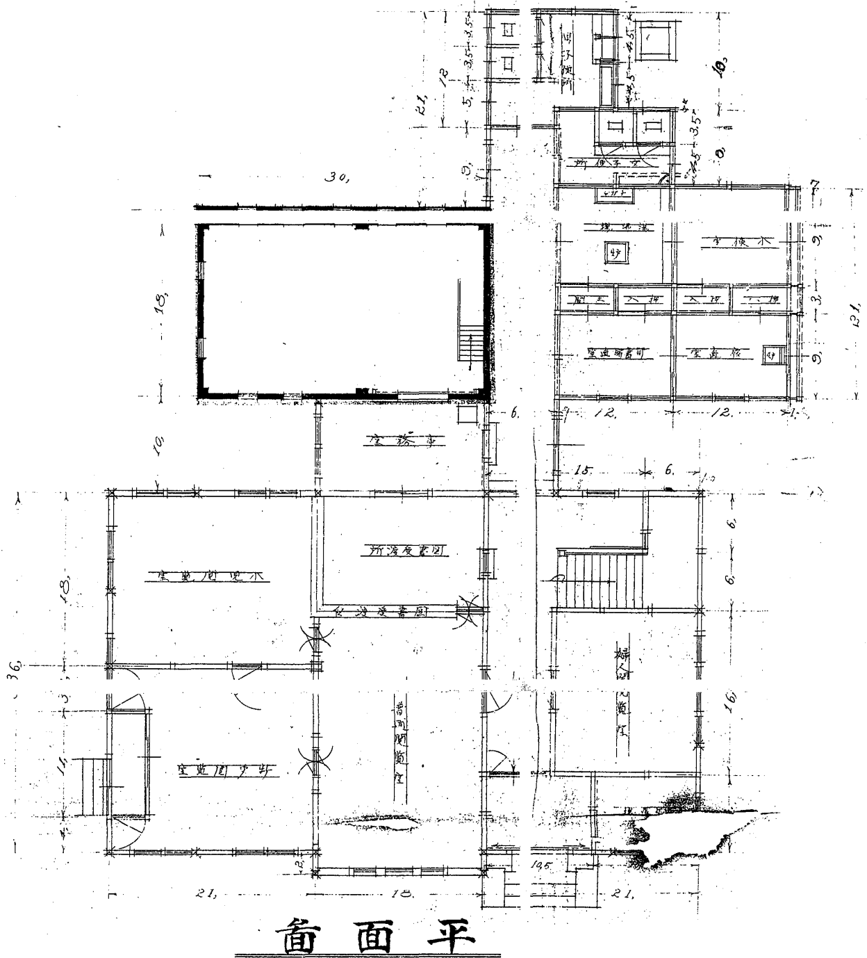
市立小樽図書館新築工事設計図 (平面図)
