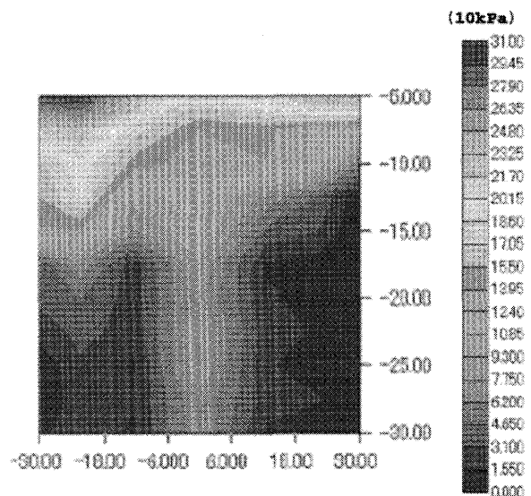
図4 コンター図(土槽内)
