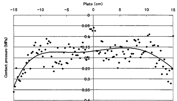
図3 載荷板の圧力分布
