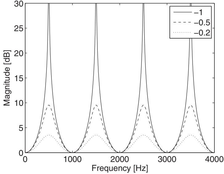
図 6：終端反射係数 r_l に対する伝達特性の変化. r_l = -1, -0.5, -0.2 , l = 17\text{cm} , c = 340\text{m/s} .
