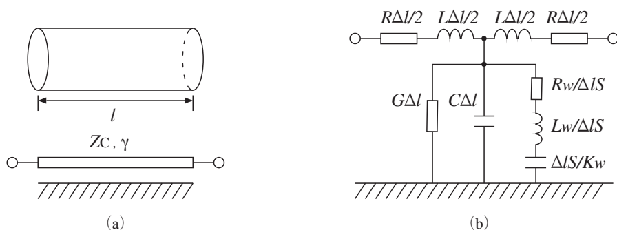
図 9 : (a) 音響管の電氣的等価回路. (b) 微小長 \Delta l の等価回路.
