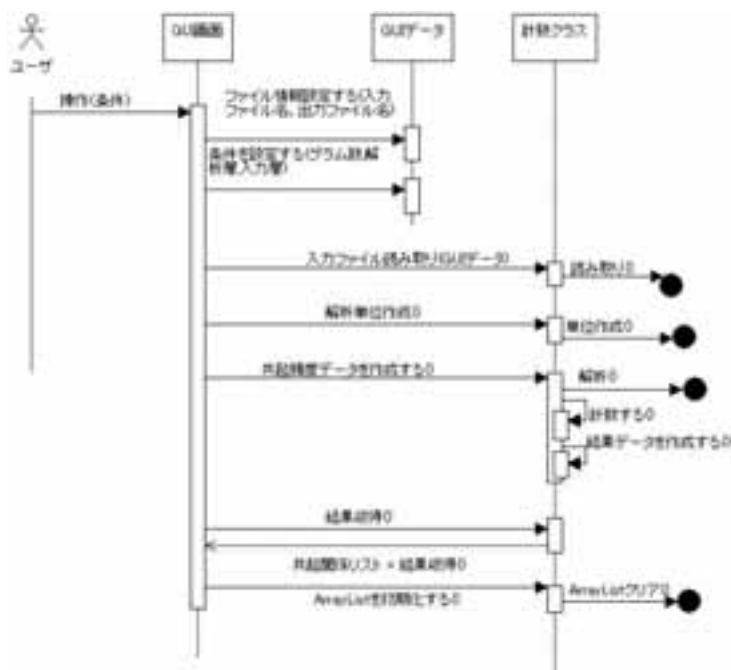
図3 層指定解析ツールのシーケンス図（トップレベル）
