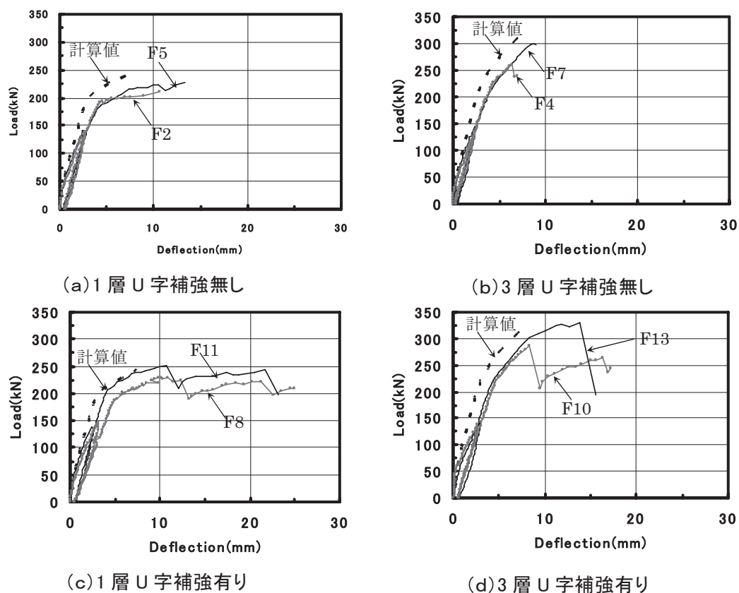
図-4 荷重-たわみ関係
