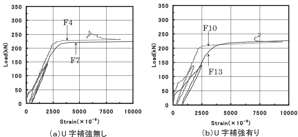
図-5 荷重-鉄筋ひずみ (3層)
