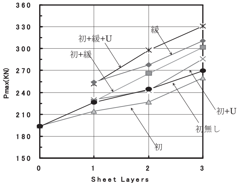
図ー3 最大荷重ーシート層数
