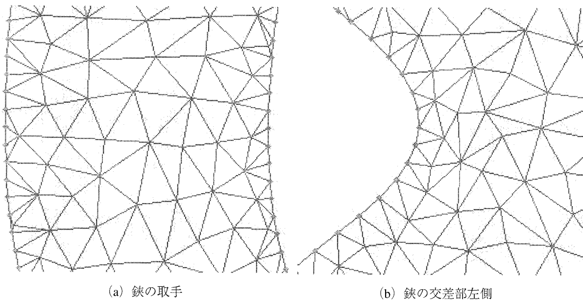
図-5 鋏最終分割形状の部分拡大
