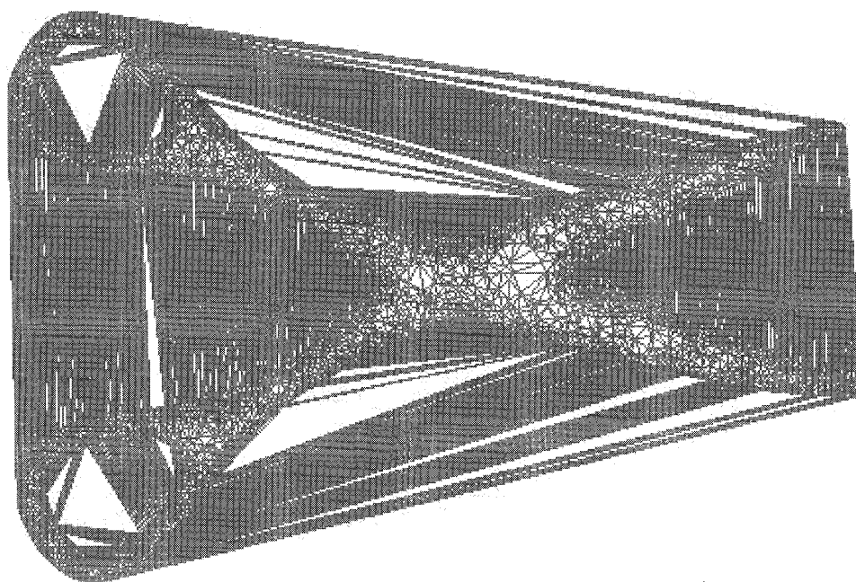
図－3 鉋のスタート時分割形状
