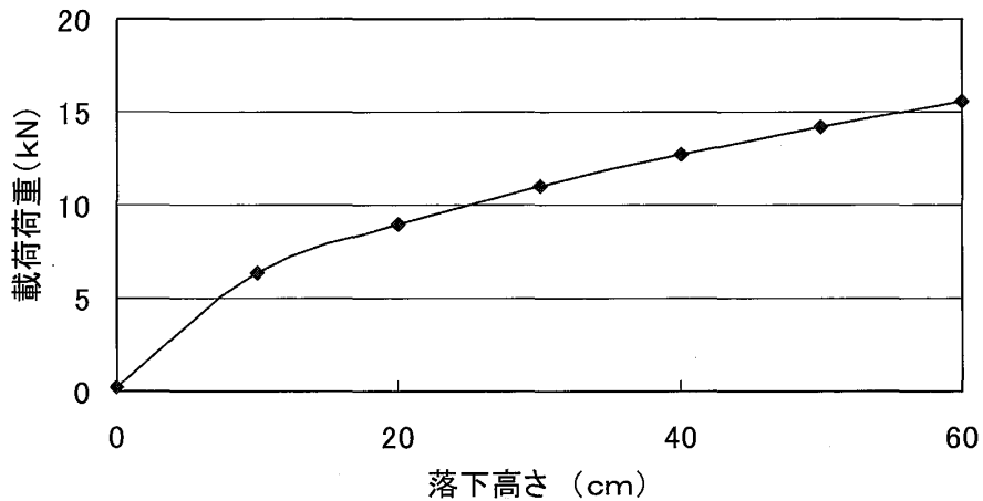
図7 重錘の落下高さと载荷荷重の関係
