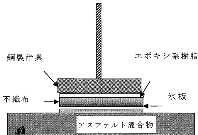
図-1 氷着強度試験の模式図
