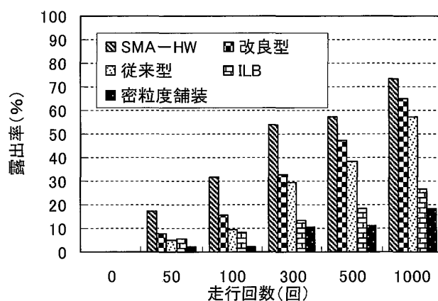
図－12 ソリッドタイヤ走行での硬圧雪路面の露出率
