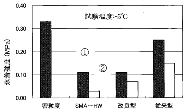
図-3 各供試体と氷着位置の違いによる氷着強度
