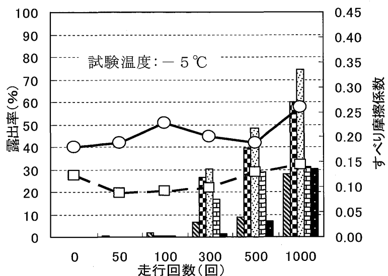
図-11 軟圧雪路面の露出率と滑り摩擦係数
