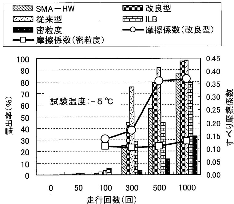
図-10 積雪路面の露出率と滑り摩擦係数
