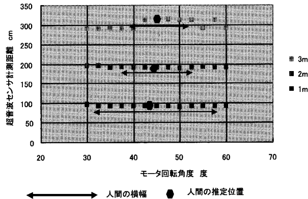
図5 焦電型赤外線センサと超音波距離センサの計測融合結果 (ロボットから45度方向1m, 2m, 3mの位置に人間が立っている状態)
