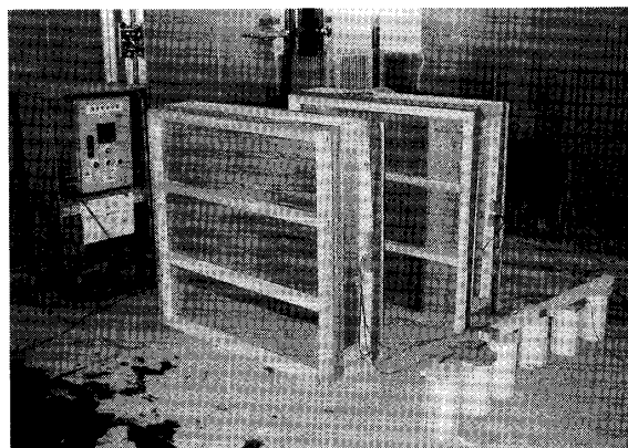
写真一 三 コンクリート打込み後の模擬試験体 型枠
