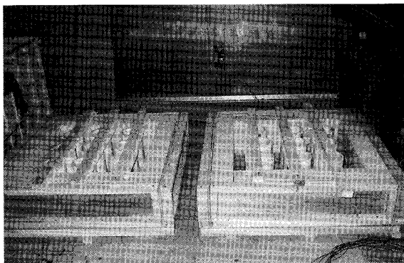
写真一 二 コンクリート打込み前の模擬試験体 型枠
