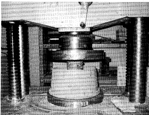
写真一8 高強度を有する供試体の圧縮強度試験 (破壊時の供試体飛散防止カバー付)
