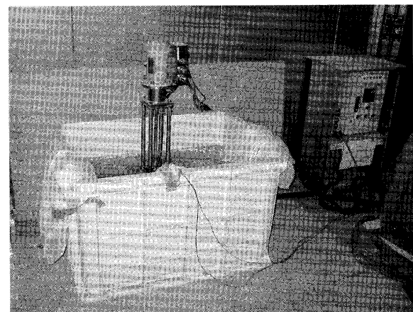
写真一 六 コンクリート供試体を定温養生装置 で養生中
