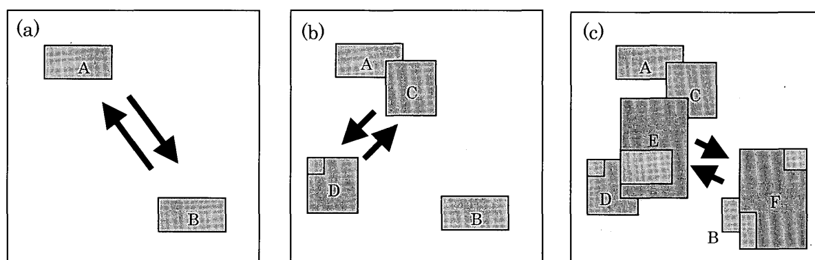
図8 多重ロッキング。(a) はA,B領域の2領域ロッキング。(b) は (a) の結果にC,D領域間の2領域ロッキングを行う2重ロッキング。(c) さらに、E,F領域の2領域ロッキングを行う3重ロッキング。
