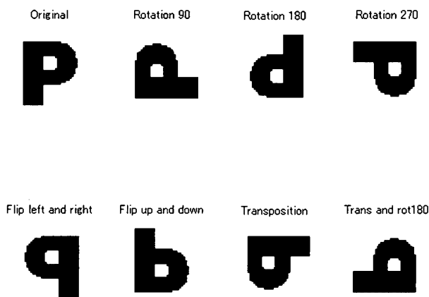
図4 単一領域ホログラムキーで用いられる演算例。
