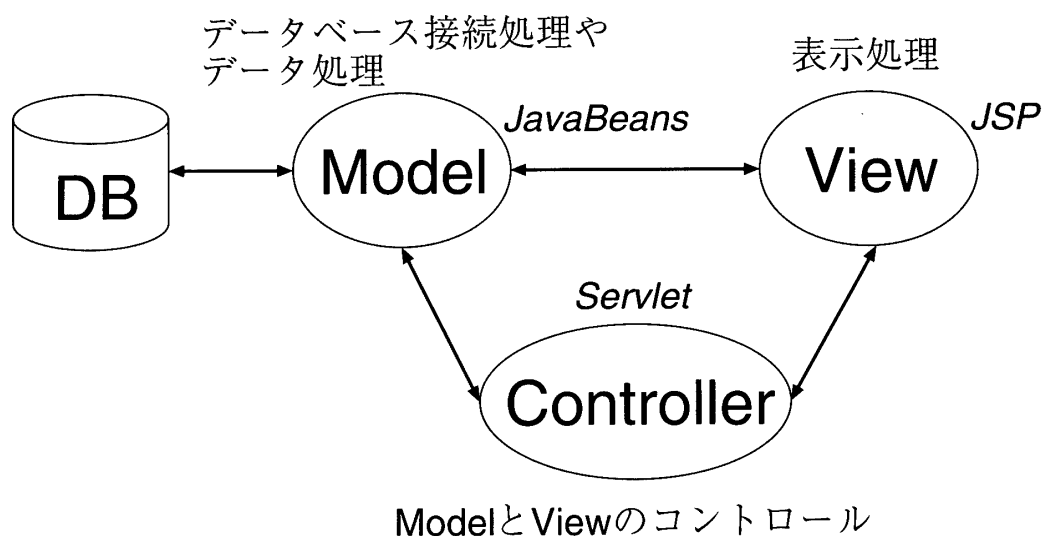
図1：MVCモデル
