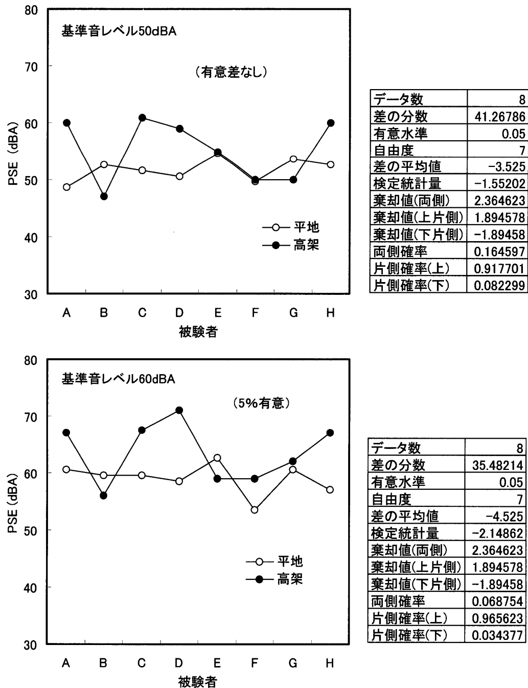
図-6 高架走行音と平地走行音の実験結果の比較
