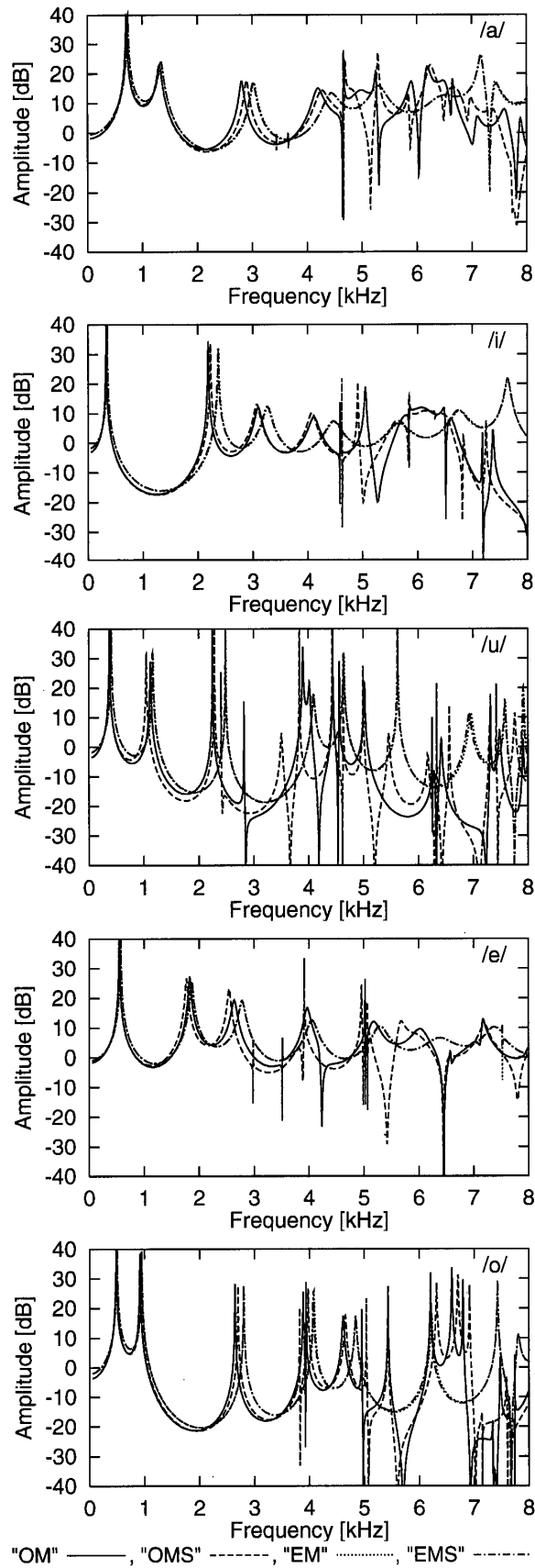
図5 声道壁を剛壁と仮定した場合の声道伝達特性(上から順に母音/a/, /i/, /u/, /e/ および/o/に対応する。図中の実線, 破線, 点線, 1点鎖線は, それぞれ OM, OMS, EM, EMS の声道伝達特性である。)
