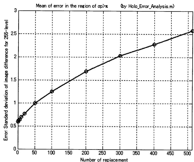
図 5 ホログラムの欠陥数の関数としての再生像の平均誤差
