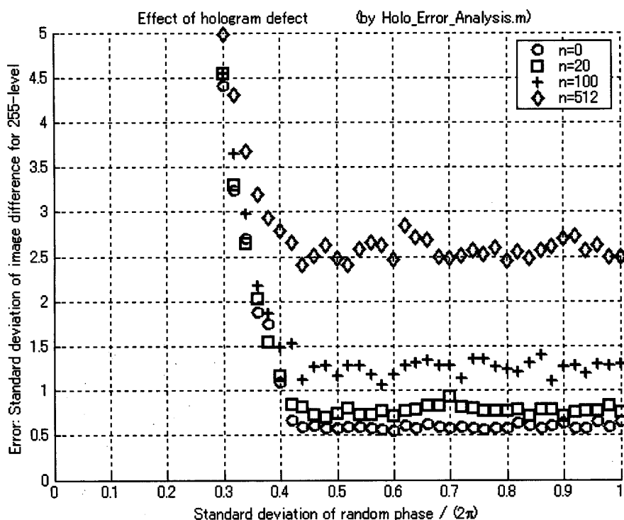
図 4 8 ビットホログラムからの再生像の誤差。横軸はランダム位相の標準偏差、縦軸は式(3)で定義される元画像と再生像の画像差の標準偏差。マーカー○はホログラム欠陥が無い場合。マーカー□, +, ◇は、それぞれ、ホログラム欠陥数 n が 20, 100, 512 の場合。
