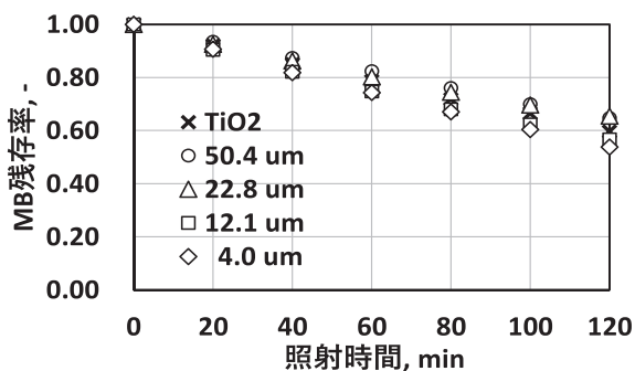
図2 有機物粒子径とメチレンブルー除去率との関係 浸漬実験。UV光源はLED（ピーク280 nm）、照射強度測定波長は254 nm、照射強度は 97 \mu\text{W}/\text{cm}^2 、 n=2 、エラーバーは最大最小値。
