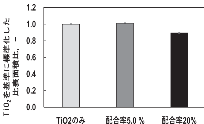
図5 \text{TiO}_2 のみを基準とした比表面積の比 \text{N}_2 ガス吸着法による細孔分布測定結果からBET法により算出, n = 3 , エラーバーは最大最小値。
