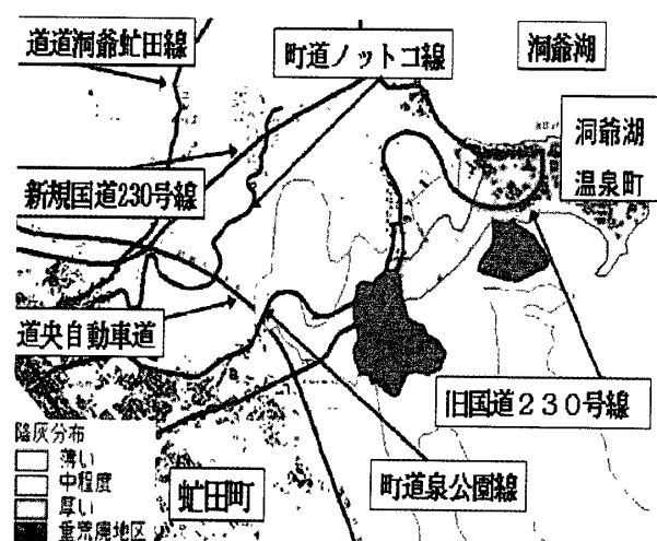
図4 降灰分布
