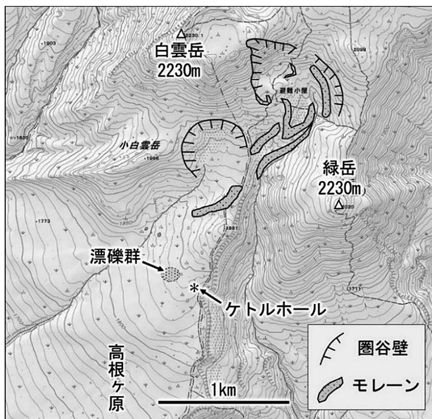
図14 白雲岳，高根ヶ原周辺の氷河地形（地理院地図を改変）
