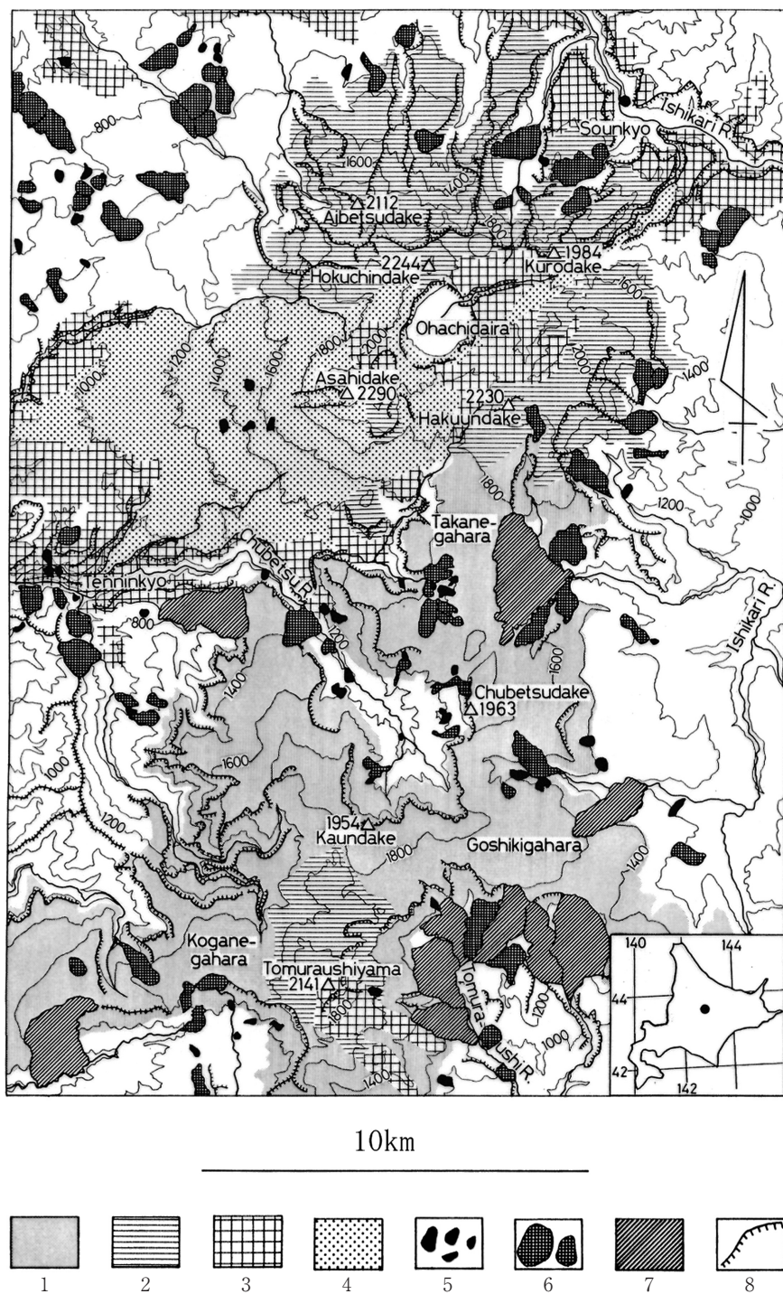
図2 大雪山地域の地質と崩壊地形分布（地質分布は国府谷ほか，1966；1968による）
