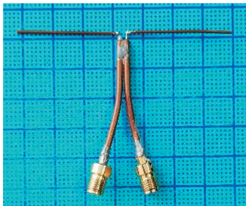
図2 セミリジッドケーブル製のジグとダイポールアンテナ
