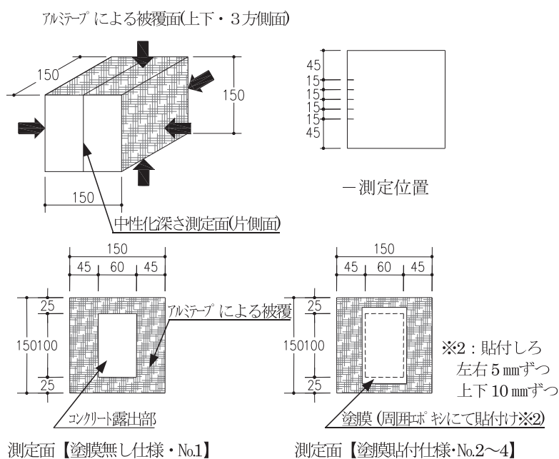
図 2 供試体概要
