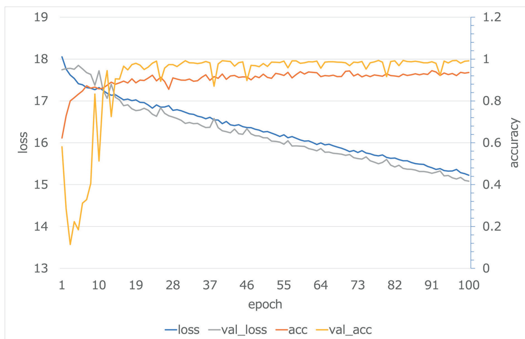
図4：学習過程
