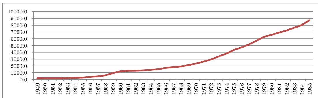
図9 1949-85年の発電設備容量の推移 単位：kW
