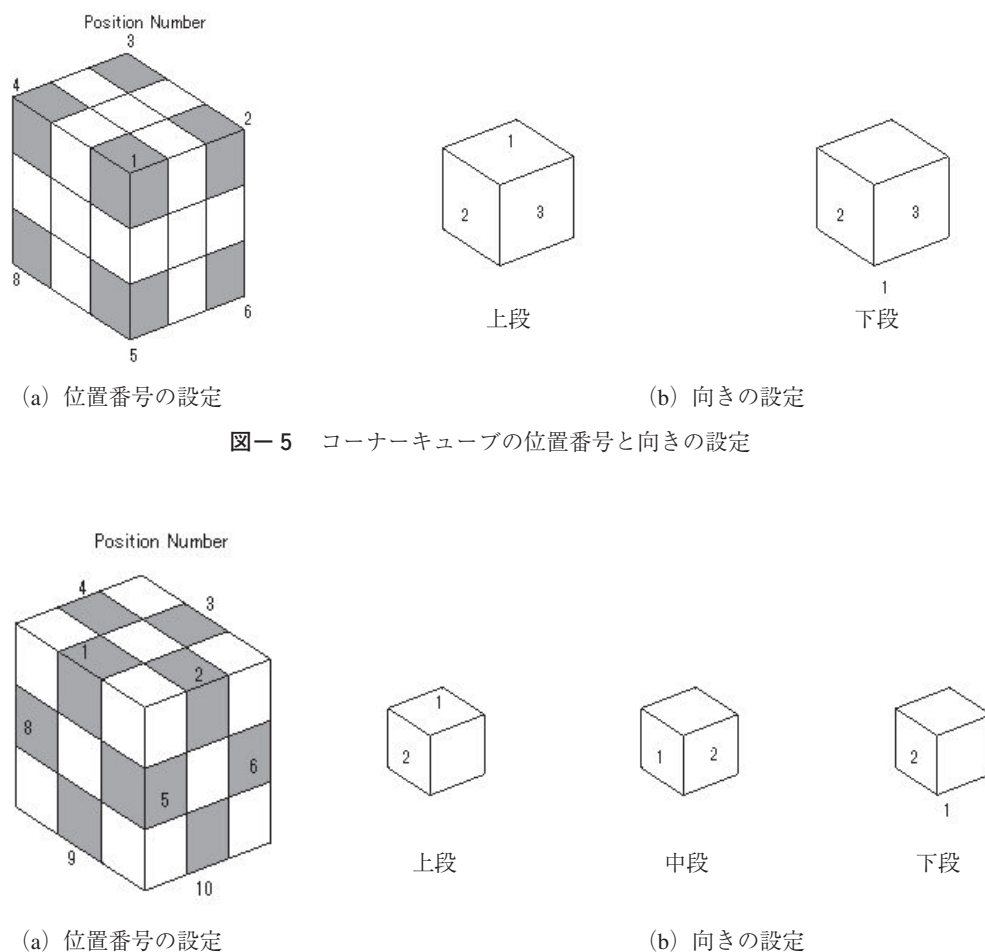
図-6 エッジキューブの位置番号と向きの設定
