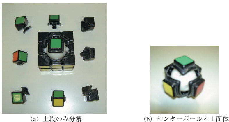
写真-1 ルービックキューブの構造
