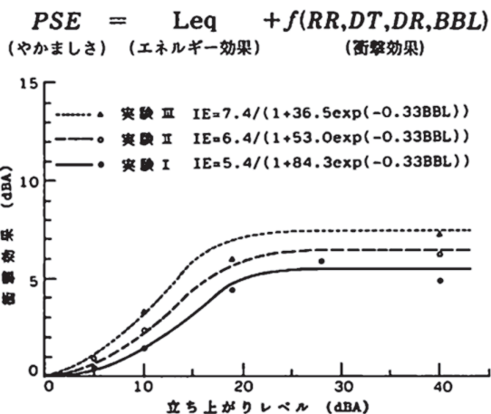
図-7 立ち上がりレベルと衝撃効果の関係
