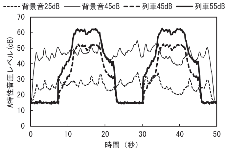
図7 背景音と試験音の波形（列車騒音の場合）
