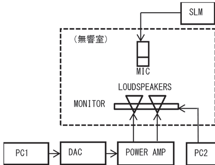
図6 実験装置のブロックダイアグラム
