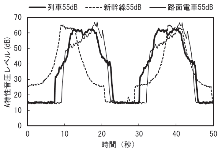
図8 各試験音の波形 (LAeq=55dBの場合)
