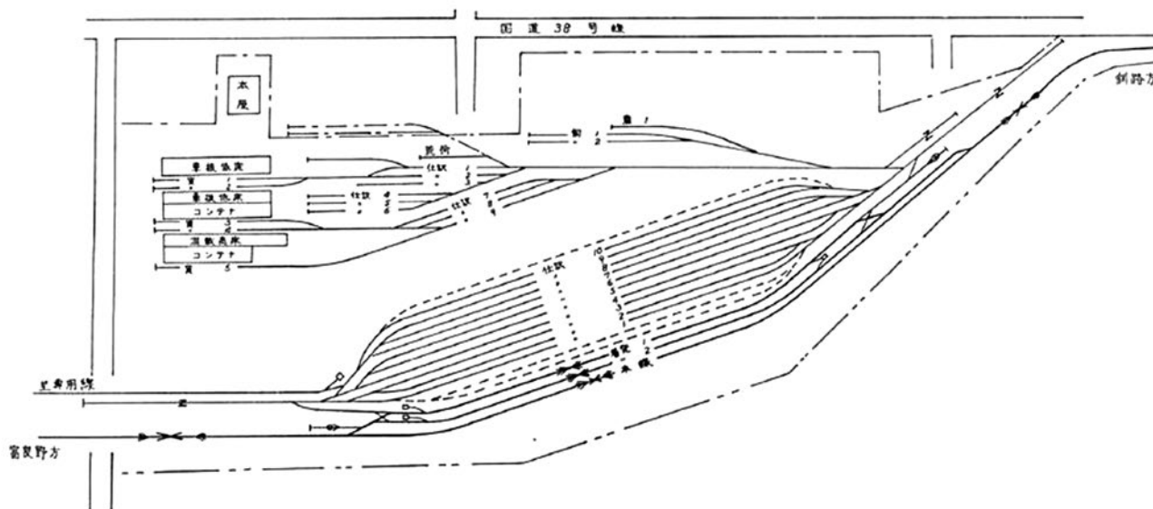
図-1 貨物ヤードの配線例（帯広貨物駅）
