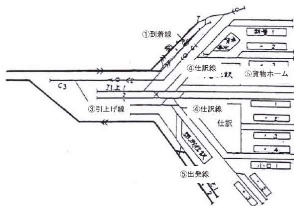
図-2 頭端式貨物駅の配線
