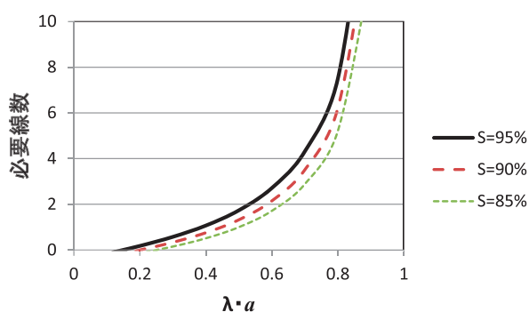
図-4 出発線の必要線数
