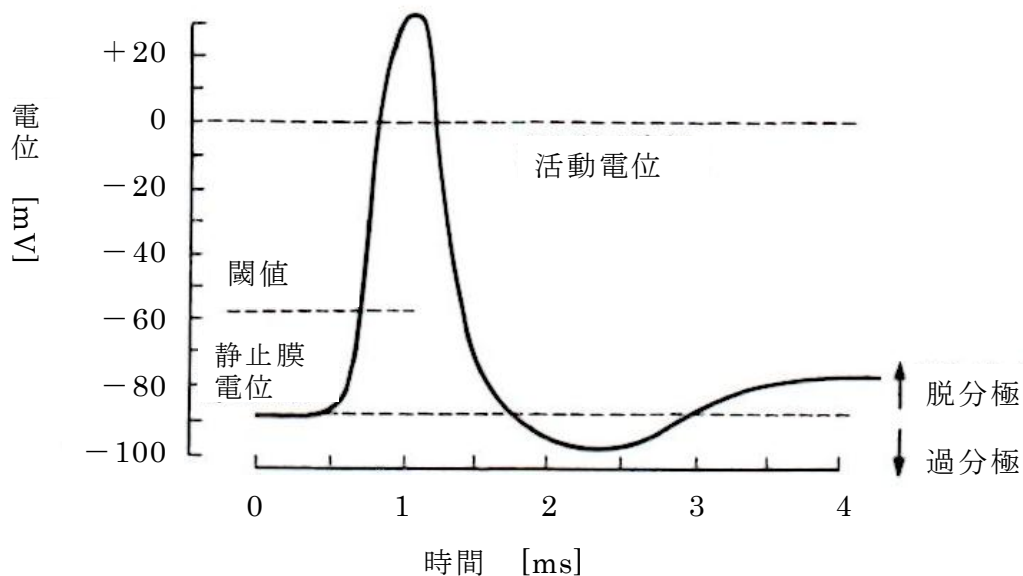
図 2.14 活動電位 [9]
