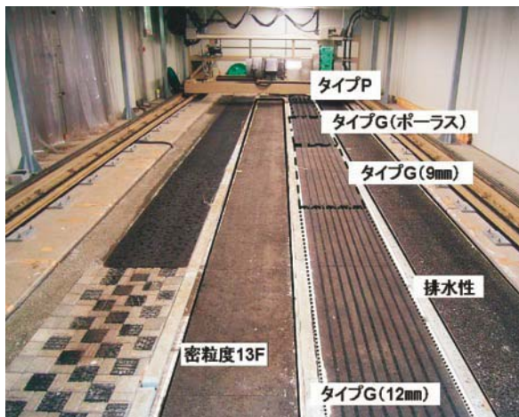
写真 2.1 走行試験装置と試験路面
