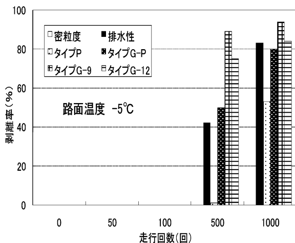
図 4.5 硬圧雪路面の雪氷剥離率
