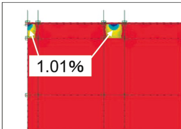
図 5.10 タイプ G-12 のひずみ
