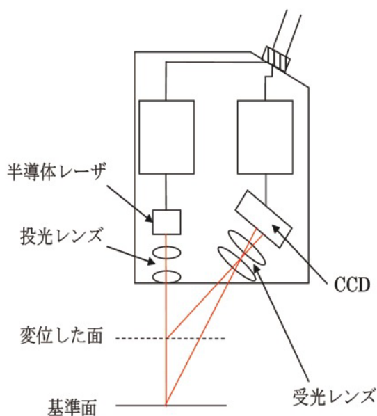
図 3.1 レーザ変位計概略図
