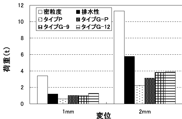
図 3.8 1 mm 変位時と 2 mm 変位時の荷重
