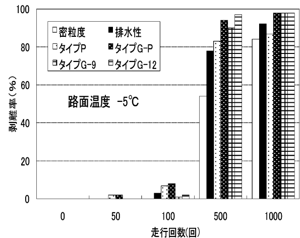
図 4.7 積雪路面の雪氷剥離率
