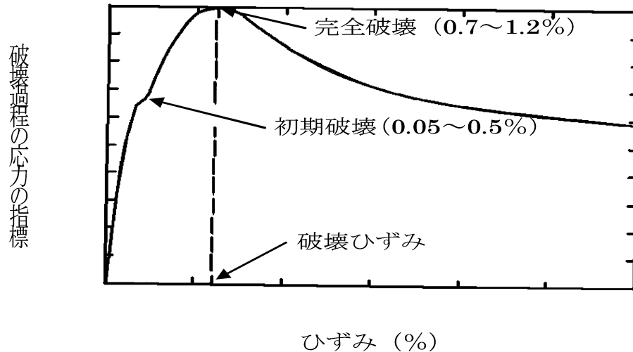
図 5.2 氷板の破壊過程 10)
