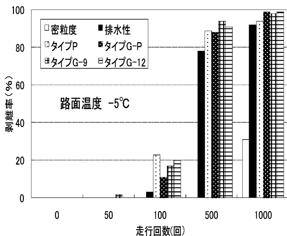
図 4.6 軟圧雪路面の雪氷剥離率
