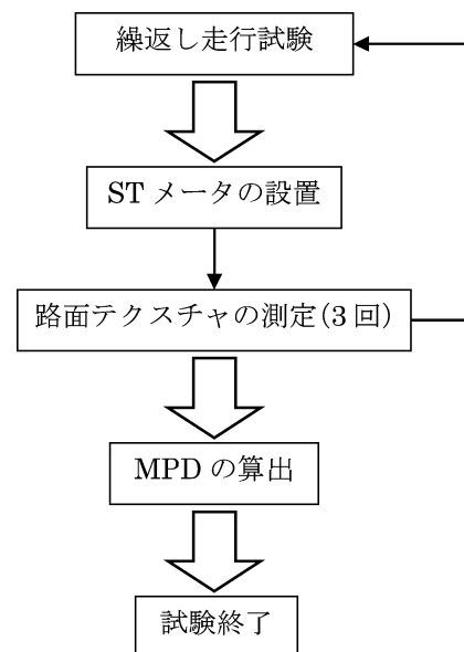
図 3.2 路面テクスチャ測定試験手順
