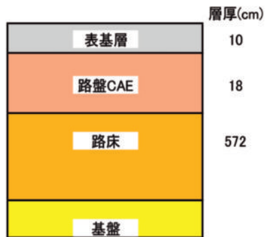
図-2 代表的な舗装断面（広島(A)）
