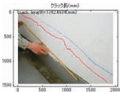
(c) ひび割れ長 (1342mm)
