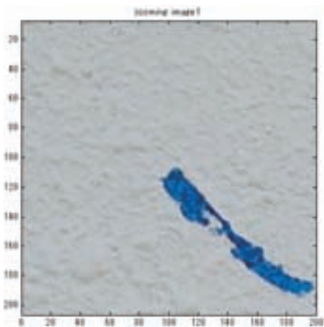
(e) ひび割れ左端点側拡大画像
