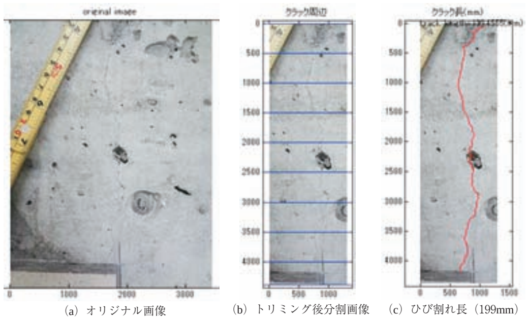
図ー 8 ケース 1 (タイル下ひび割れ, 有効画素数4608×3456pixel)
