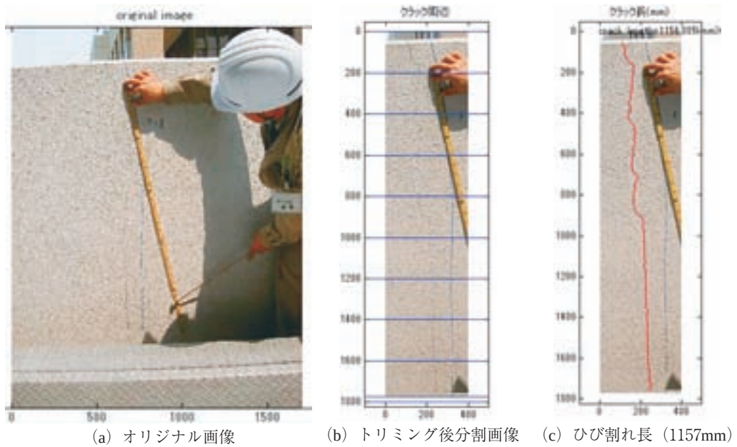
図-6 ケース1 (有効画素数2304×1704pixel)
