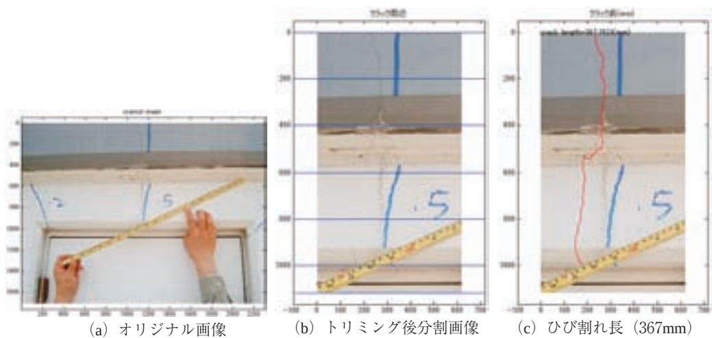
図-11 外壁面に凹凸を有する不適当な算定ケース (有効画素数2304×1704pixel)
