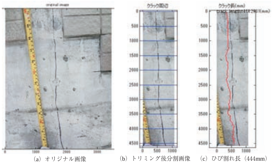
図-7 ケース5 (タイル下ひび割れ, 有効画素数4608×3456pixel)
