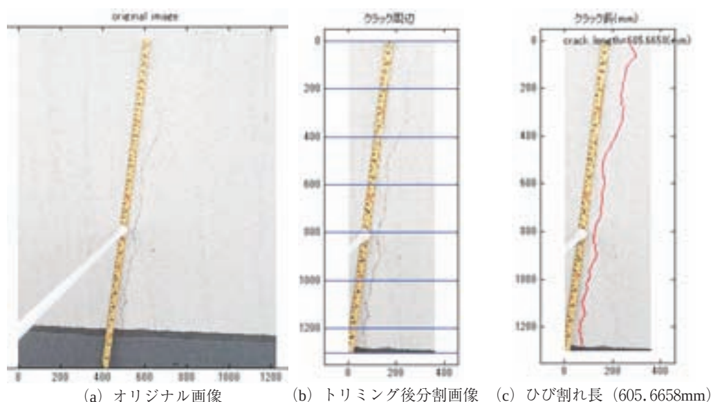
図-12 統計処理実施ひび割れサンプル (有効画素数2304×1704pixel)
