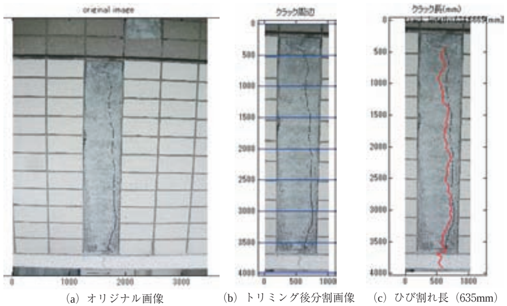
図ー 9 ケース 4 (タイル下ひび割れ, 有効画素数4608×3456pixel)
