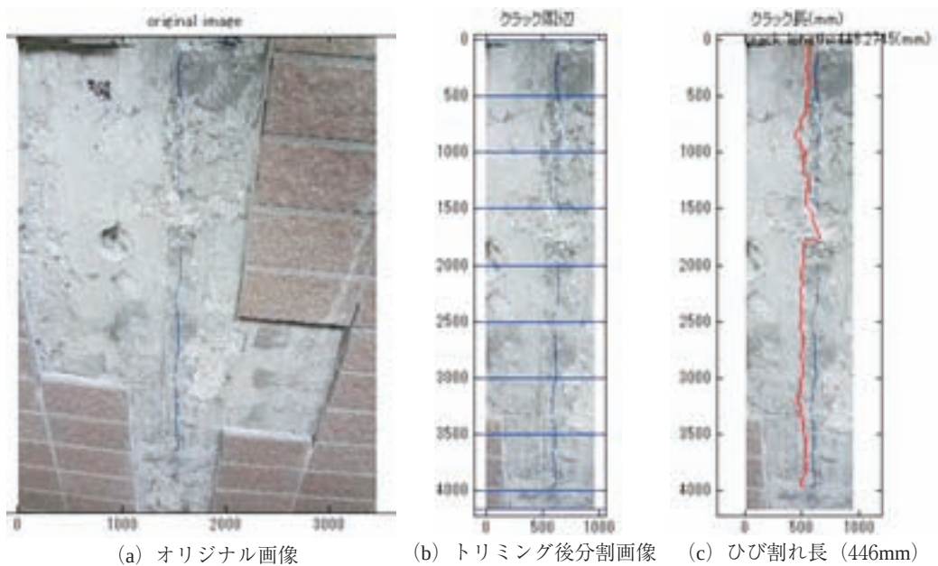
図-10 ケース 4, 7 (タイル下ひび割れ, 有効画素数4608×3456pixel)
