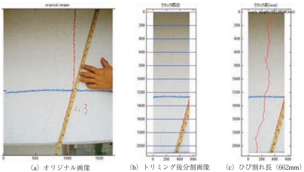
図-2 ケース1 (有効画素数2304×1704pixel)
