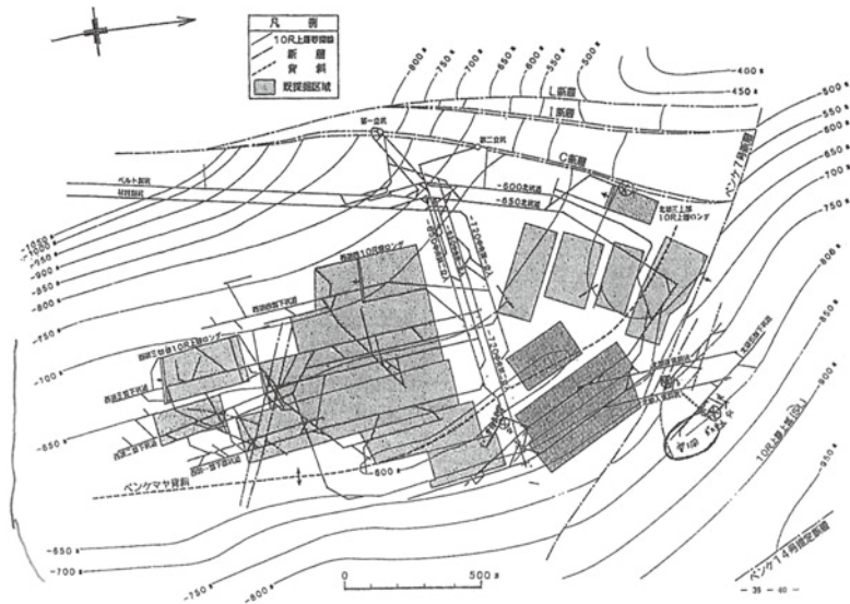
図表 43 夕張新炭鉱炭層深度図
