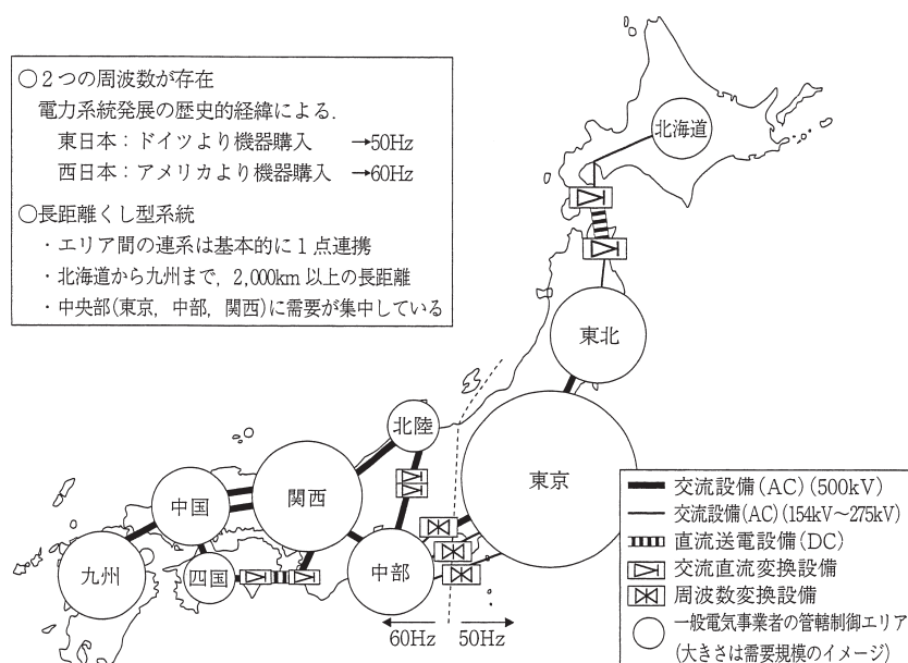
図1 電力系統
