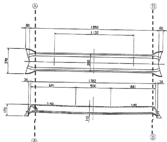
図-2 使用した鉄まくらぎ
