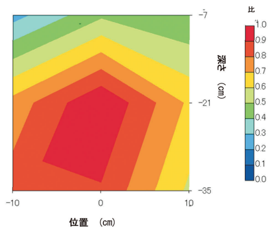
図-7 2 値化による比較コンター図（木まくらぎ）
