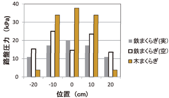
図-13 路盤圧力の分布（横断方向）
