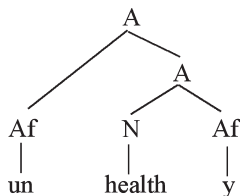
図 4.8 unhealthy の構造
