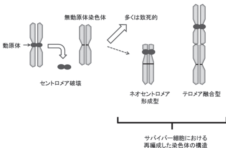
図4. 分裂酵母のセントロメア破壊による2種類の染色体再編成現象
