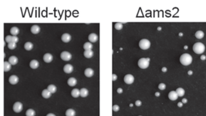
図6．分裂酵母Ams2破壊株のコロニー形成能
