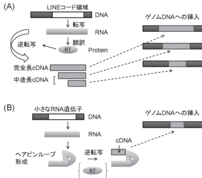
図 2. LINEおよびSINEファミリーの構造とゲノムへの侵入の仕方 4)
