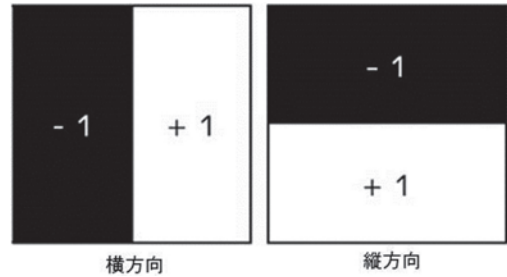
図6 Haar wavelet
