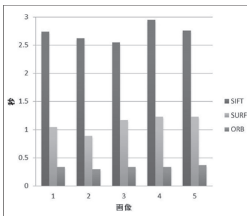
図9 計算時間
