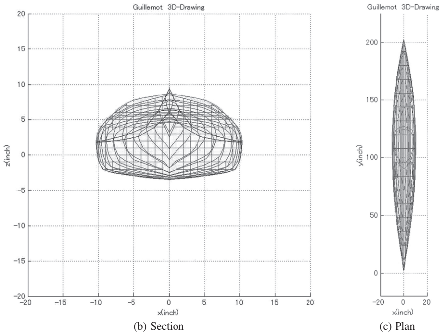
図-1 船体形状
