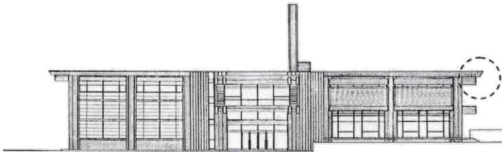
東側立面図*4
