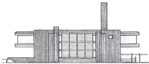
東側立面図*2
