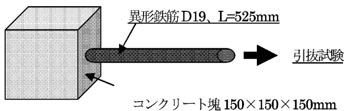
図2. 引抜試験概要図
