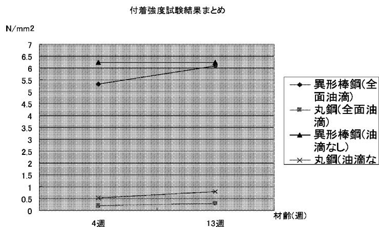
図5. 付着強度試験結果 (まとめ)
