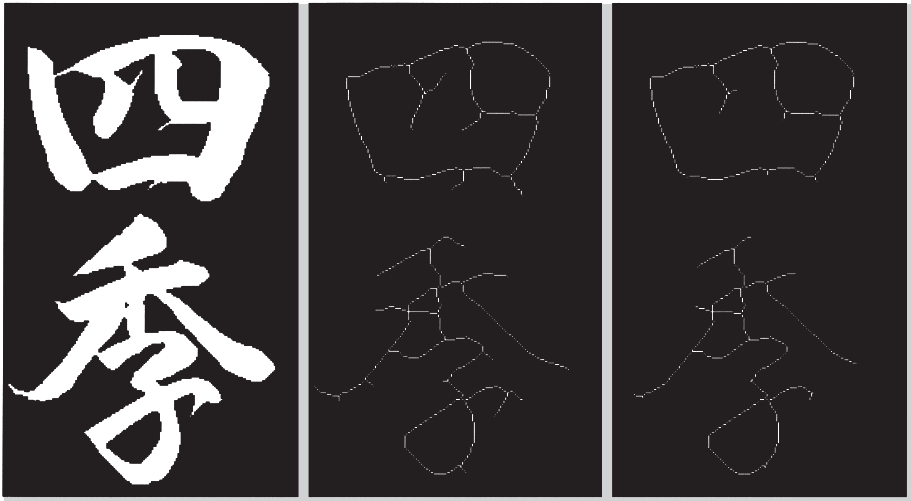
図12 (左)入力2値画像, (中)細線化された画像, (右)ヒゲ削減処理後の細線化画像(削減処理回数10).
