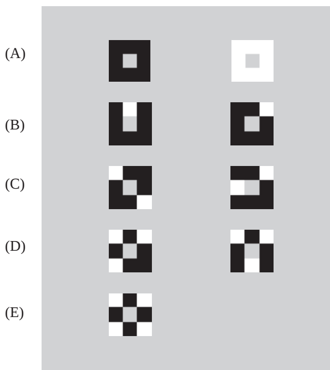
図7 連結数と注目画素の役割（注目画素が白の場合）.
