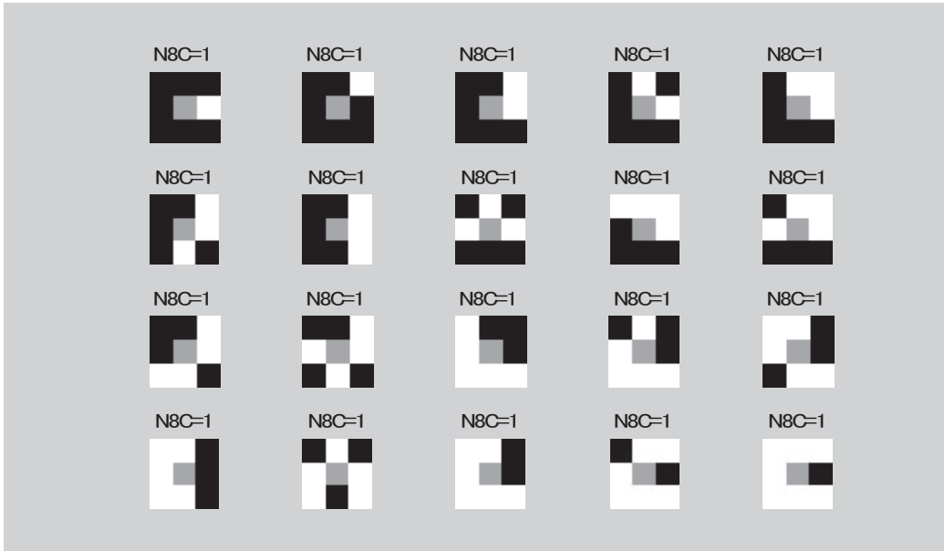
図 4 連結数 N_c^8 = 1 の 8 近傍画素パターン．注目画素が白でも黒でも 8 近傍連結の意味で白の連結成分は一つである．
