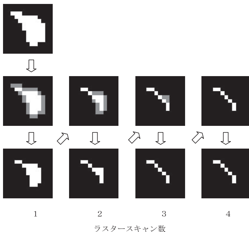
図10 細線化の処理過程．左上が入力画像で白の領域が細線化の対象．中段のグレーの画素が削除できる境界画素．下段はそれらを削除した結果．この処理をラスタースキャンごとに繰り返す．
