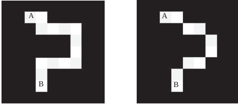
図2 画素Aから画素Bまでの4近傍連結（左）と8近傍連結（右）．黒い部分が0、白い部分が1．
