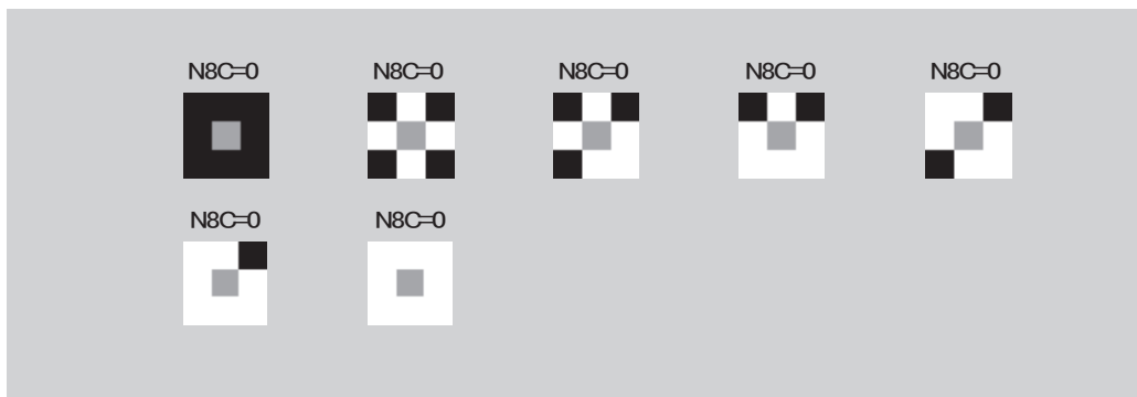
図3 連結数 N_c^8 = 0 の8近傍画素パターン．0か1である中央の着目画素はグレーで表示している．
