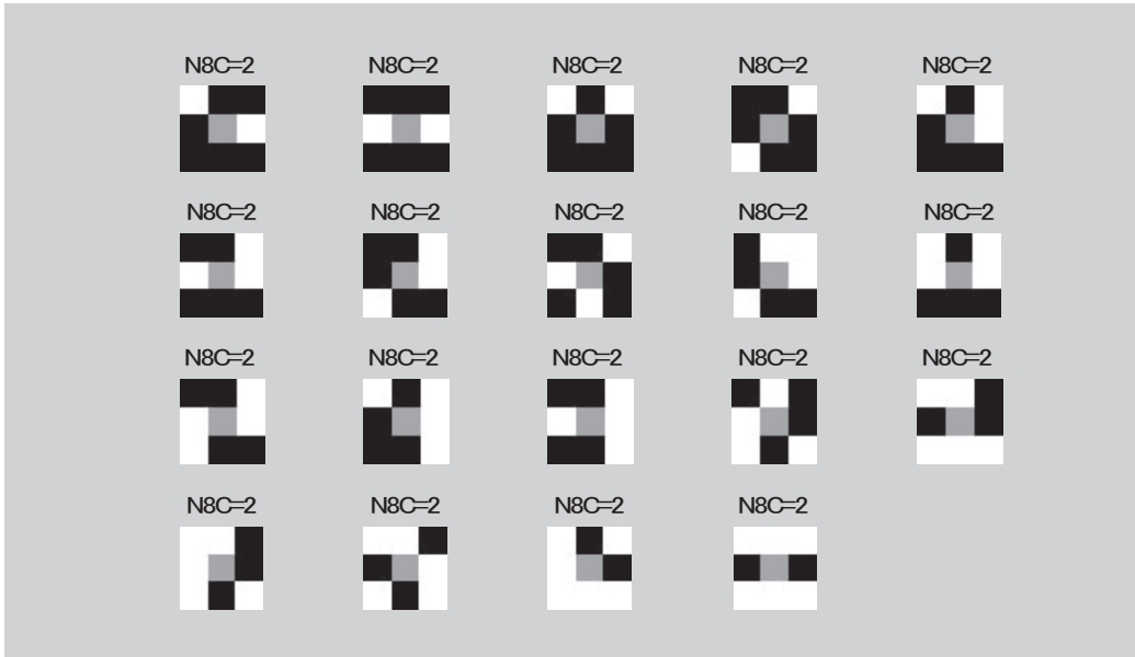
図 5 連結数 N_c^8 = 2 の 8 近傍画素パターン．中央の注目画素が白であれば，白の連結成分は一つであるが，黒であれば白の連結成分は二つに分かれる．
