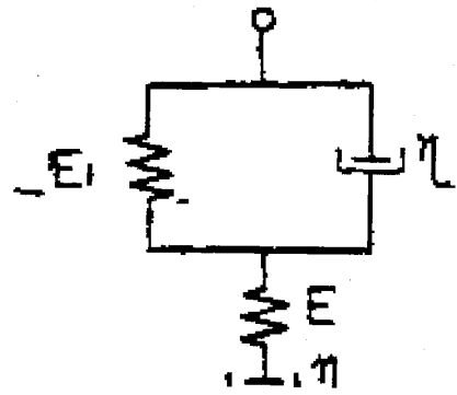
図7 Maxwell-Kalvin モデル
