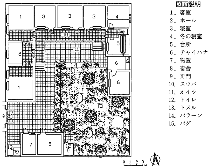
図8 n字形平面 (13) 建設1960年代
