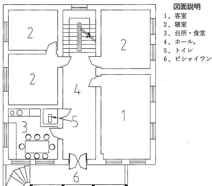
図9 ロシア式建築の影響を受けた民家の平面 (14) 建設1990年代
