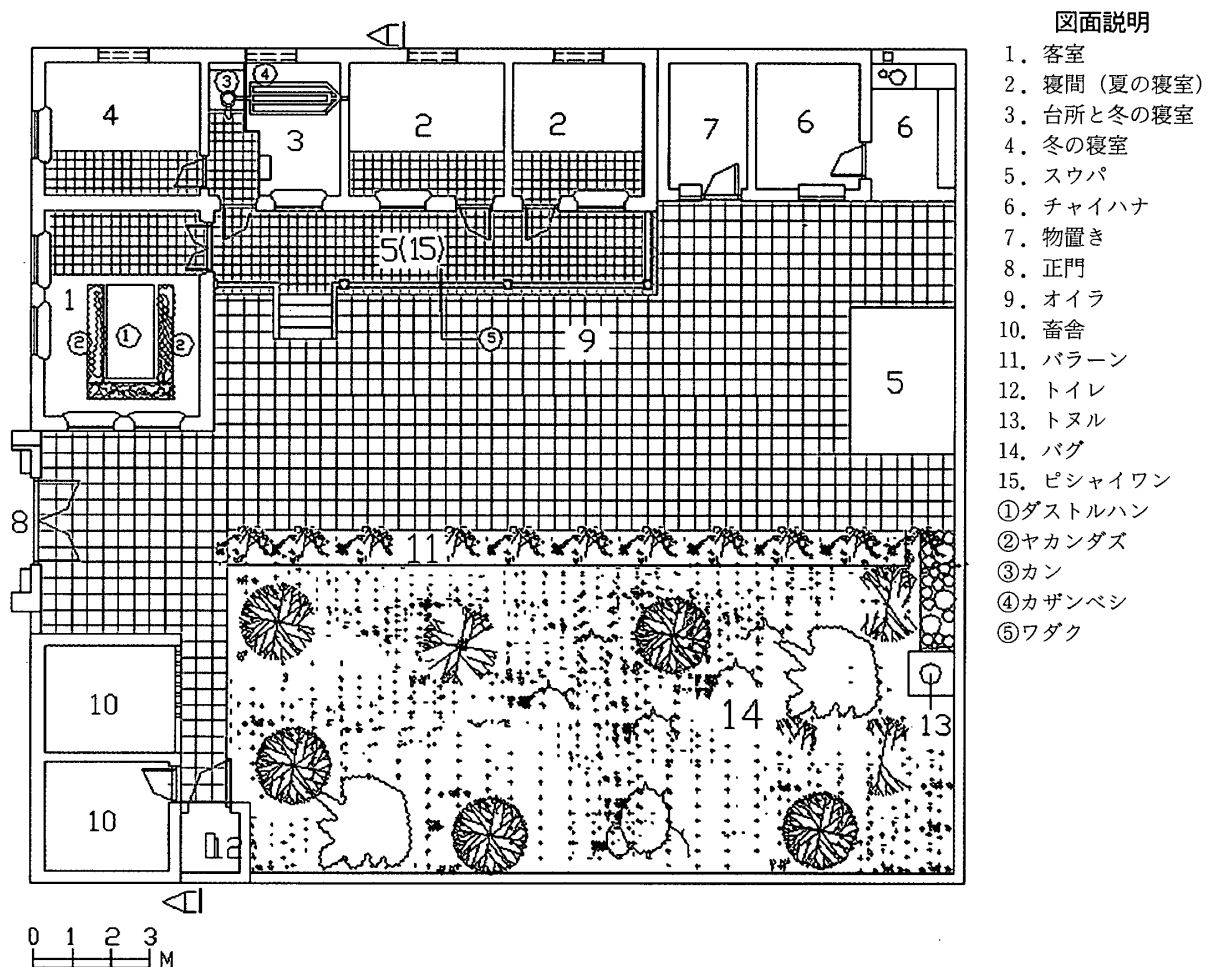
図2 イリの民家の一般的平面（建設年1920年代） (7)
